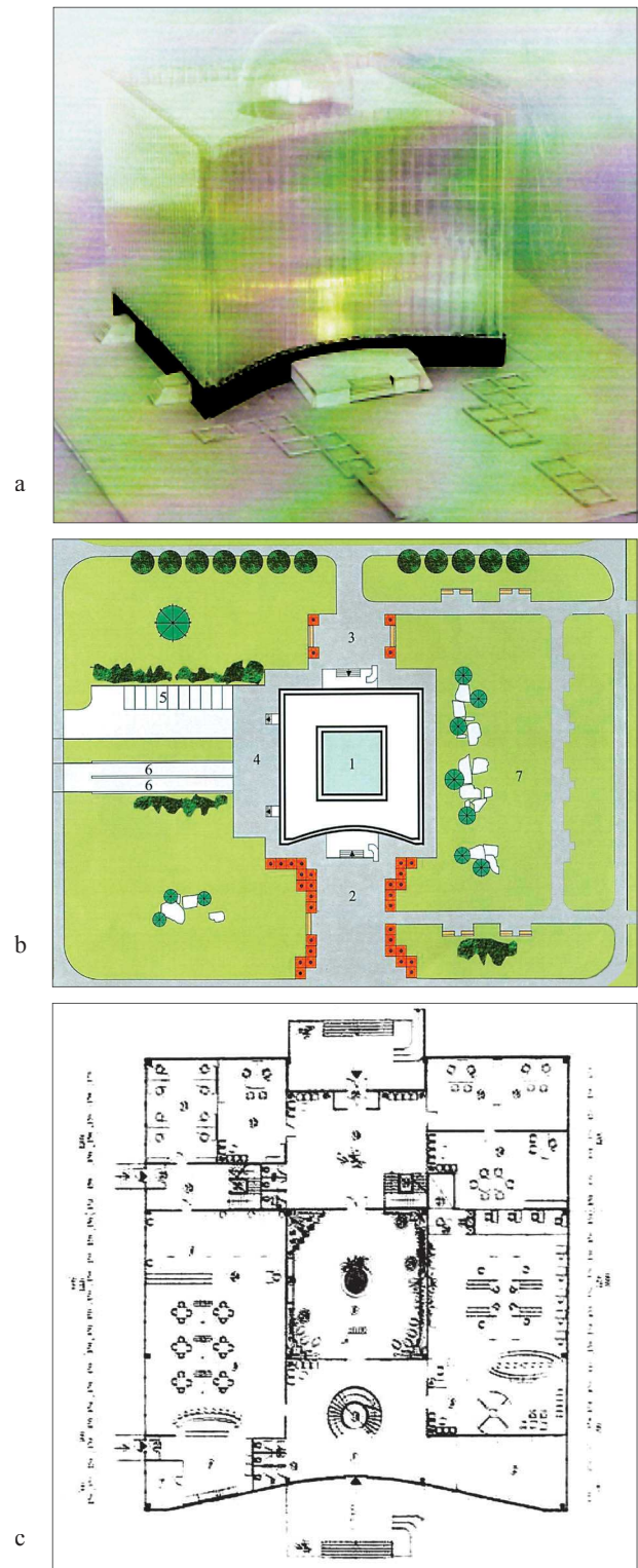
12 pav. Konceptinis viešosios bibliotekos Vilniuje projektas (autoriai K. Jakovlevas-Mateckis ir L. Kostinaitė, 2003 m.):
